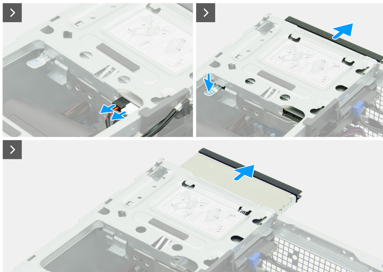
Rysunek 37. Wymontowywanie napędu optycznego
