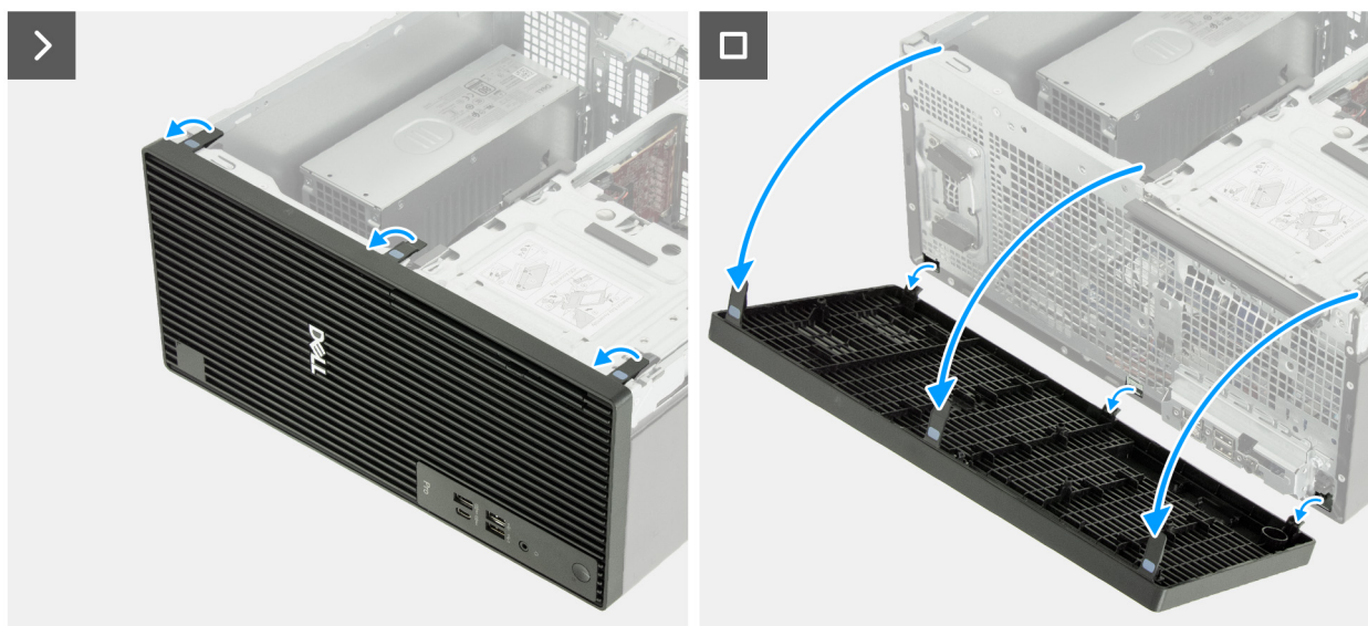
Rysunek 22. Wymontowywanie pokrywy przedniej
