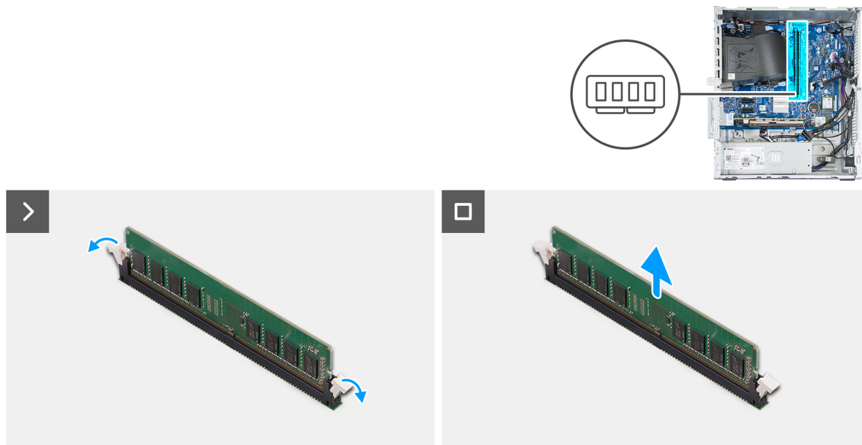
Rysunek 26. Wymontowywanie modułów pamięci
