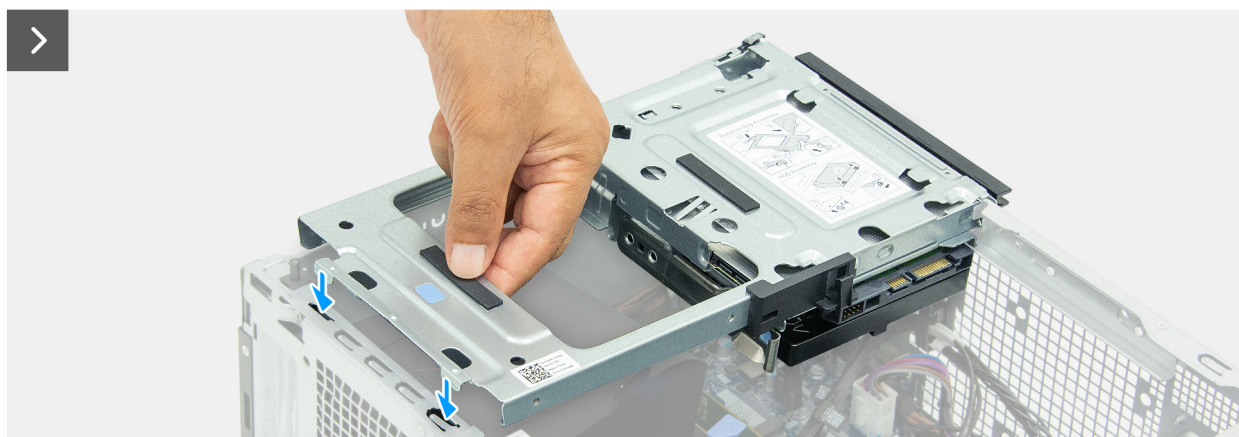
Rysunek 43. Instalowanie wnęki napędu
