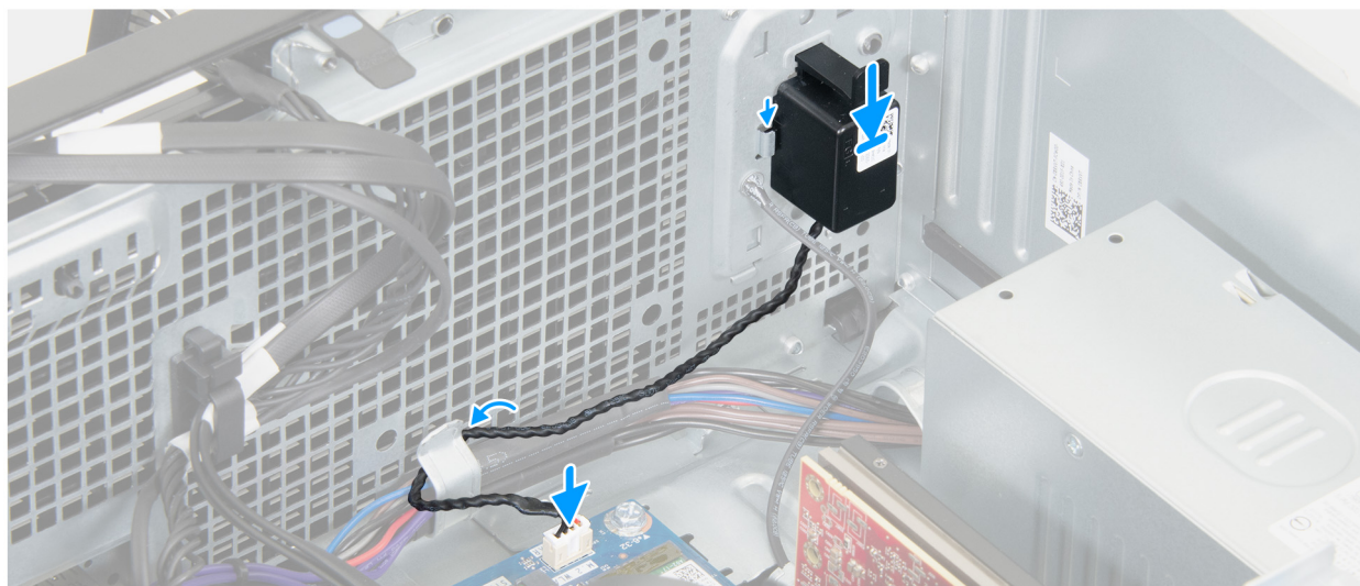
Rysunek 25. Instalowanie głośnika wewnętrznego
