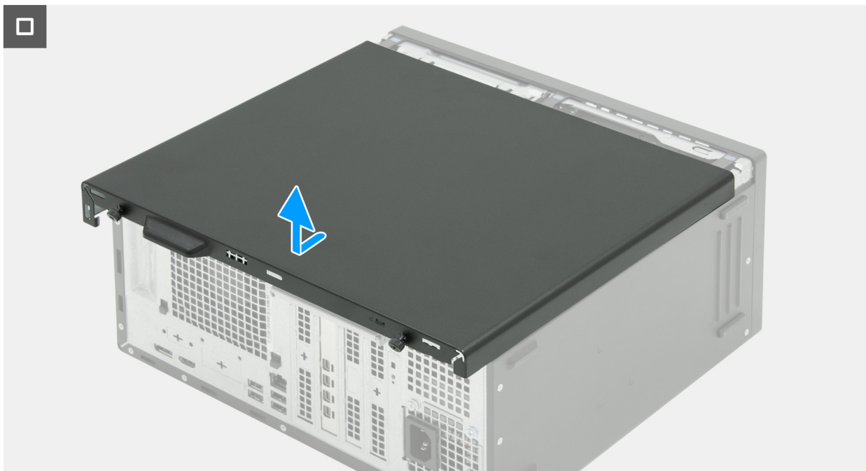
Rysunek 13. Wymontowywanie lewej pokrywy bocznej
