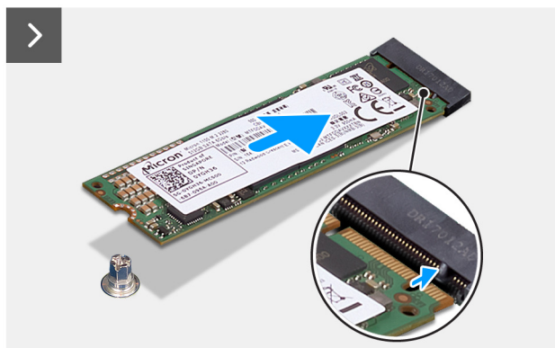
Rysunek 31. Instalowanie dysku SSD M.2 2280
