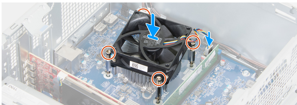
Rysunek 66. Instalowanie zestawu wentylatora i radiatora procesora
