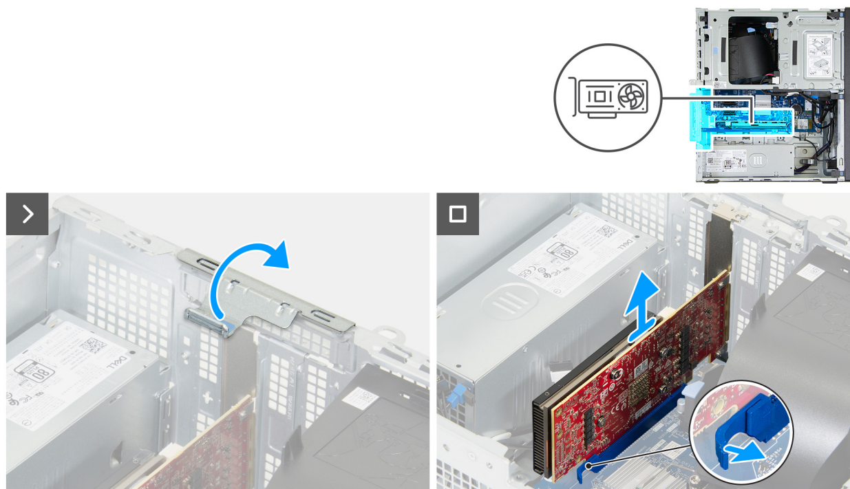
Rysunek 33. Wymontowywanie karty graficznej
