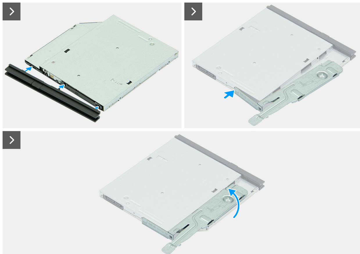
Rysunek 39. Instalowanie napędu optycznego
