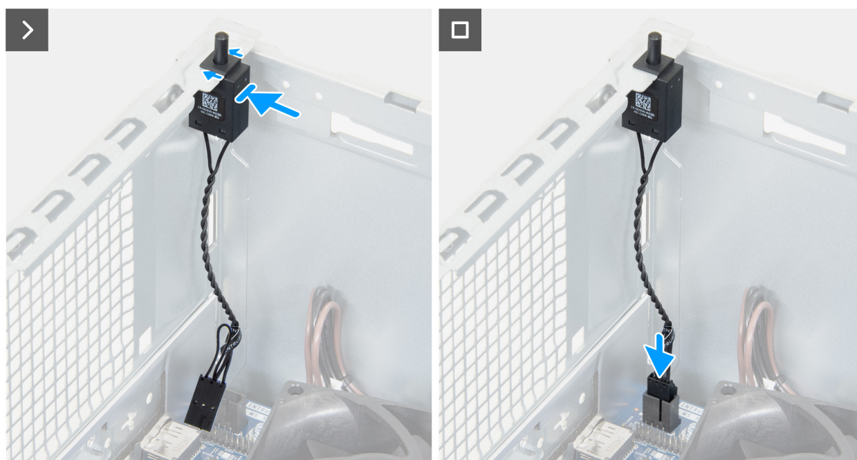
Rysunek 48. Instalowanie czujnika otwarcia obudowy
