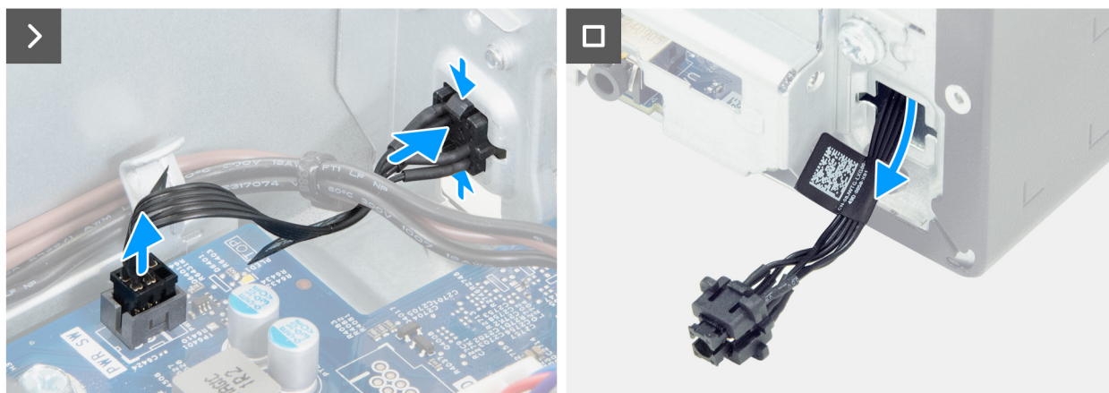
Rysunek 49. Wymontowywanie przycisku zasilania
