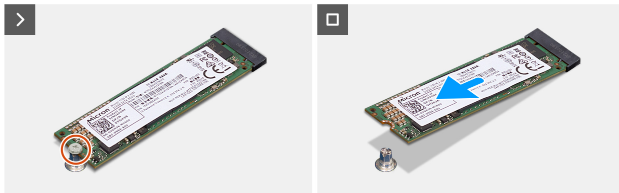
Rysunek 30. Wymontowywanie dysku SSD M.2 2280
