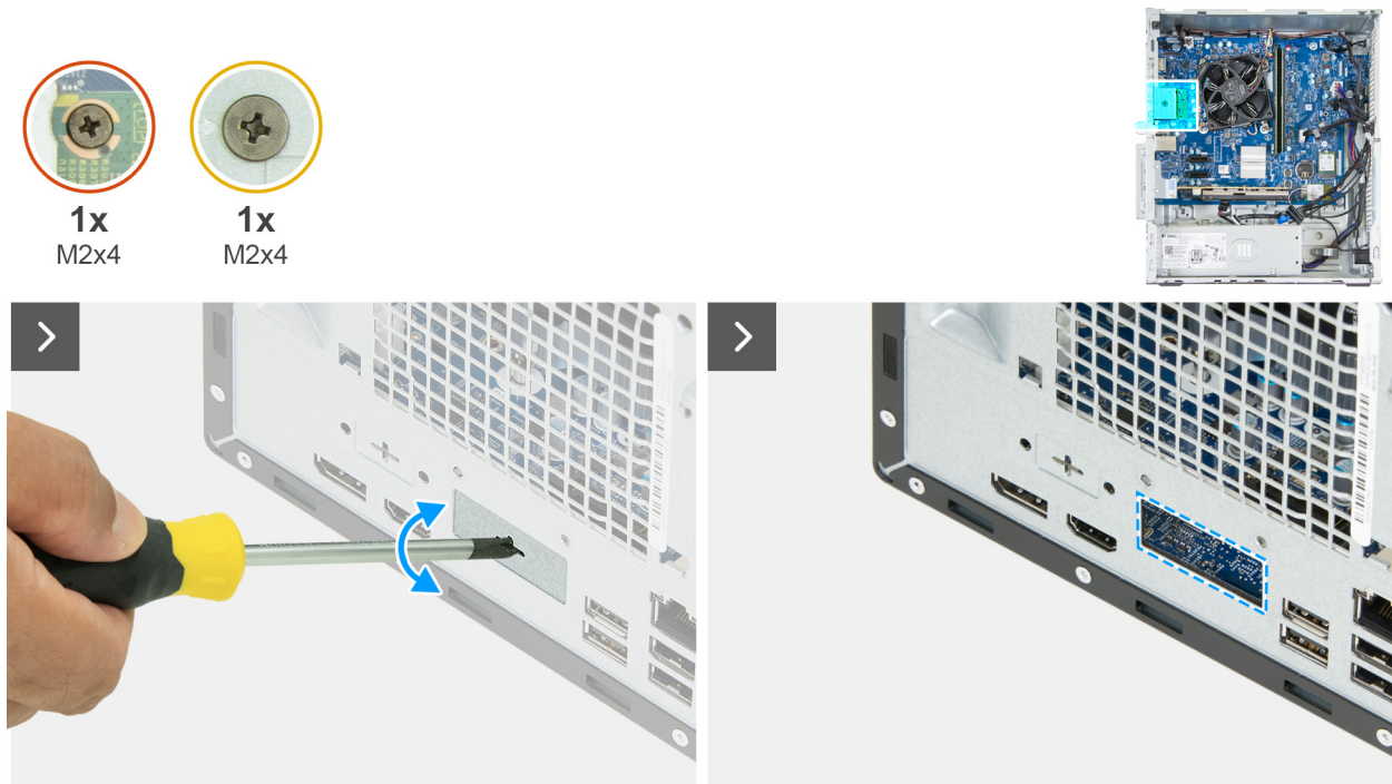
Rysunek 54. Instalowanie modułu portu opcjonalnego
