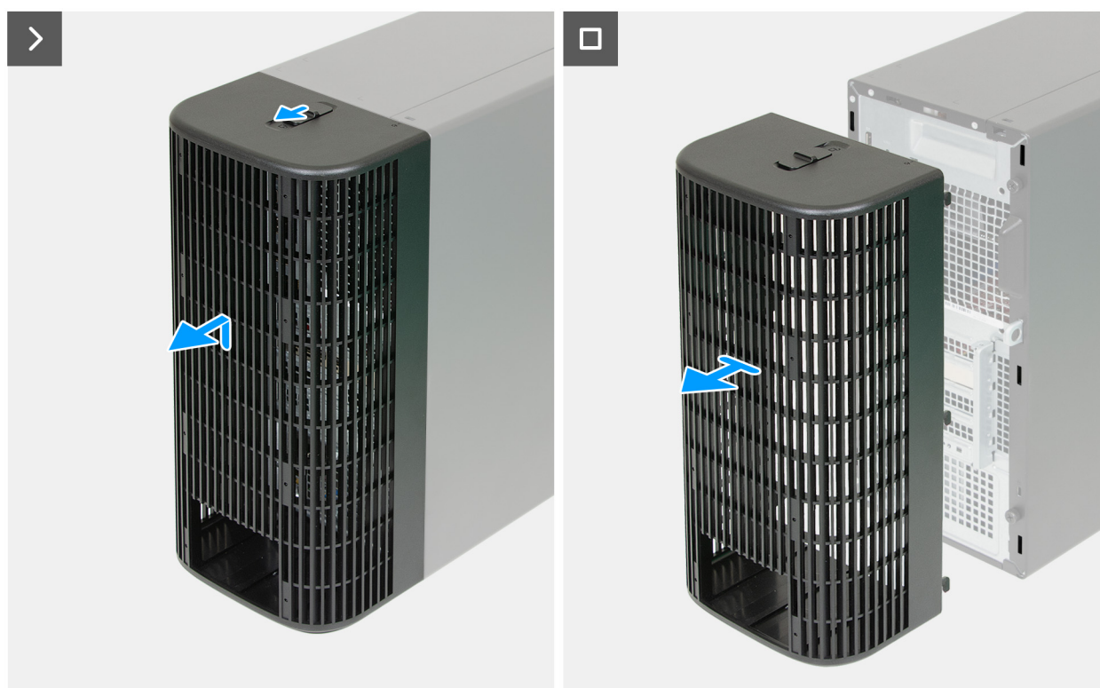
Rysunek 10. Wymontowywanie osłony kabli
