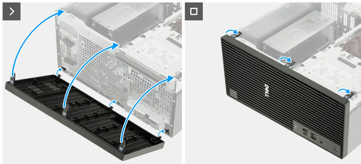
Rysunek 23. Instalowanie pokrywy przedniej
