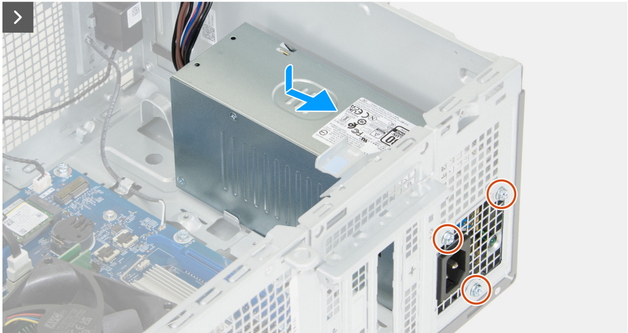
Rysunek 63. Instalowanie zasilacza
