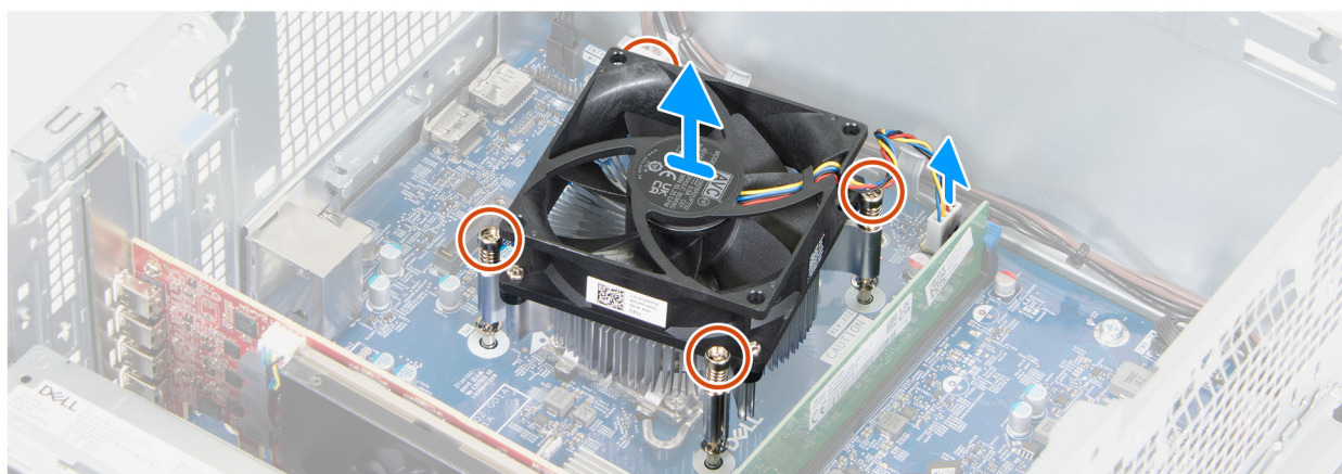
Rysunek 65. Wymontowywanie zestawu wentylatora i radiatora procesora
