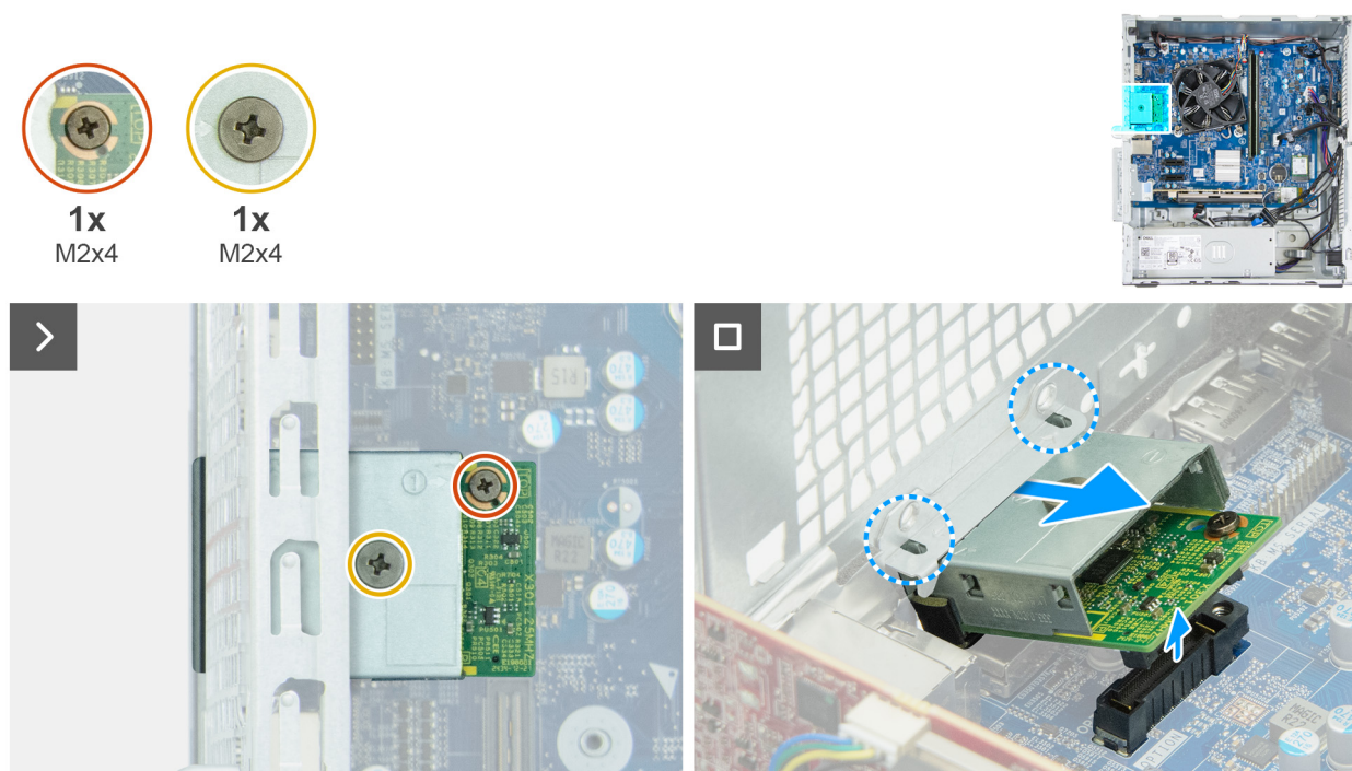
Rysunek 53. Wymontowywanie modułu portu opcjonalnego
