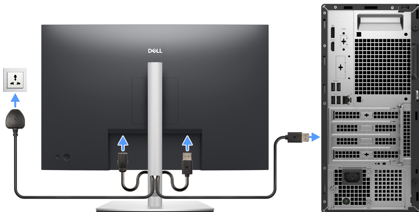
Rysunek 6. Podłączenie wyświetlacza
