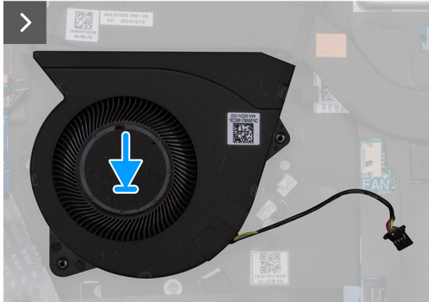
Figure 23. Installing the fan
